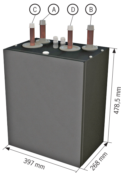
Jäähdytysmoduuli PT1000/Legend
